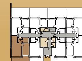
Rzut Parteru
